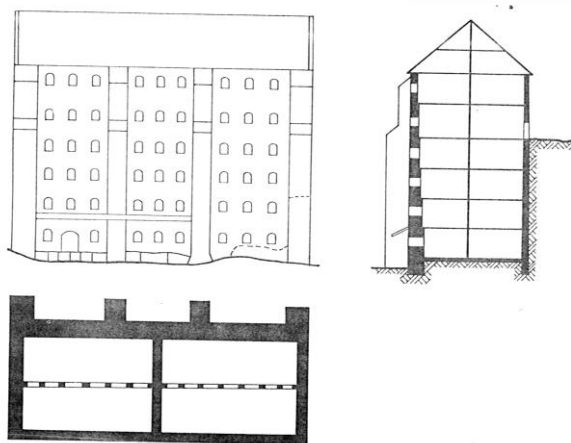
71. Spichrz gotycki z XIV w. w Grudziądzu o typowych wysmukłych szkarpach, wg rys. Z. Radackiego. Wcięcie od strony uliczki Spichrzem ponieważ 5 kondygnacji. Widoczna rytna do spustu ziarna.
