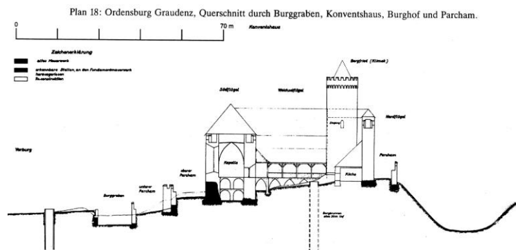
Przekrój pionowy domu konwentu na osi północ – południe. Za: H. Jacobi. Die Ausgrabungsergebnisse der Deutschordenburgen Graudenz und Roggenhausen.
