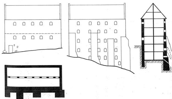
70. Spichrz gotycki z XIV w. w Grudziądzu, wg rys. Z. Radackiego. Charakterystyczna dla Grudziądza grubość muru zewnętrznego. Typowy podłużny podział wnętrza, występujący również w Kazimierzu (Gdańsk zerwał z tym podziałem usuwocześniając konstrukcję spichrza).
