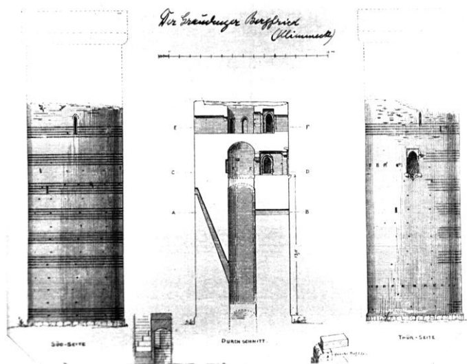
Rysunek techniczny wieży Klimek z końca XIX w. Zdjęcie ze zbiorów Muzeum w Grudziądzu
