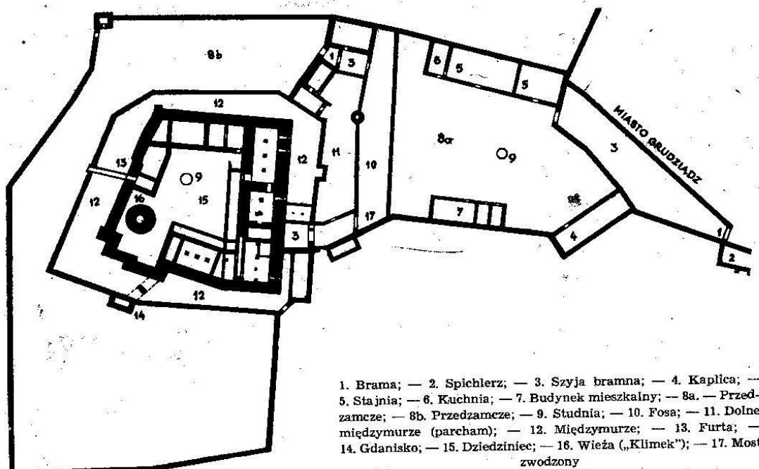
Ryc. 3. Zamek w Grudziądzu. Rekonstrukcja fundamentów i piwnic na podstawie badań z l. 1941–42
