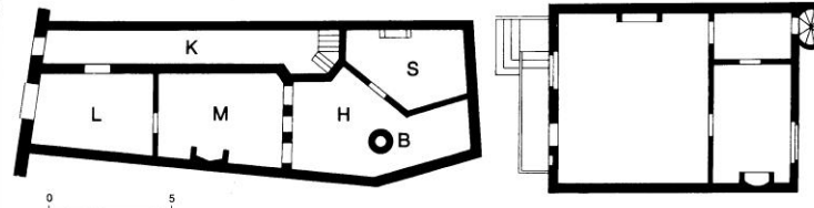
Włoskie, średniowieczne domy mieszkalne. Po lewej: XII w. (por. Cluny, 351*). K – korytarz, L – sklep, M – magazyn, H – dziedziniec ze studnią (B), S – stajnia. Po prawej: lepiej wykorzystana powierzchnia mieszkalna poprzez dobudowę schodów od zewnątrz i krótszy, możliwy do zamieszkania korytarz.
